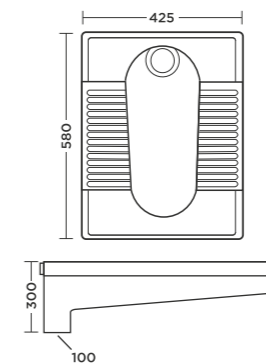
OSP - 063 | ORISSA PAN 23"
