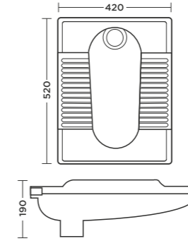
CTP - 061 | C . T . PAN 20"
