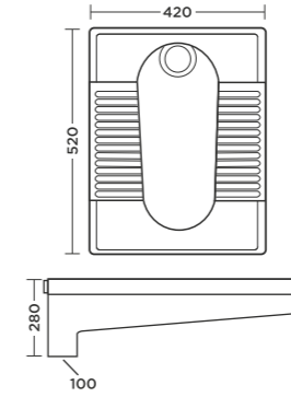
ORS - 062 | ORISSA PAN 20"
